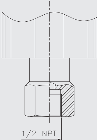
SMT2003 B
